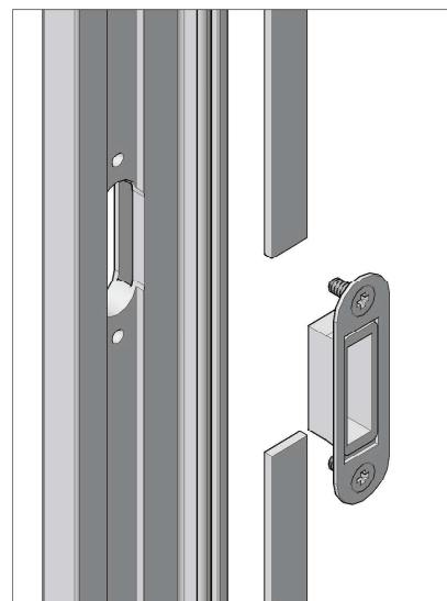
Incontro Easy-fix a doppia regolazione per serratura Magnetica Easy-fix plate for magnetic lock with double regulation
