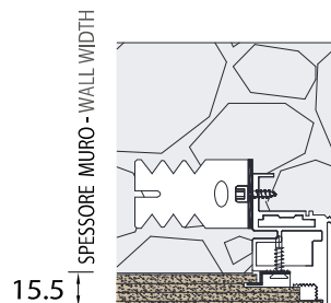
Aggancio boiserie su muratura Boiserie hanging on brickwall
