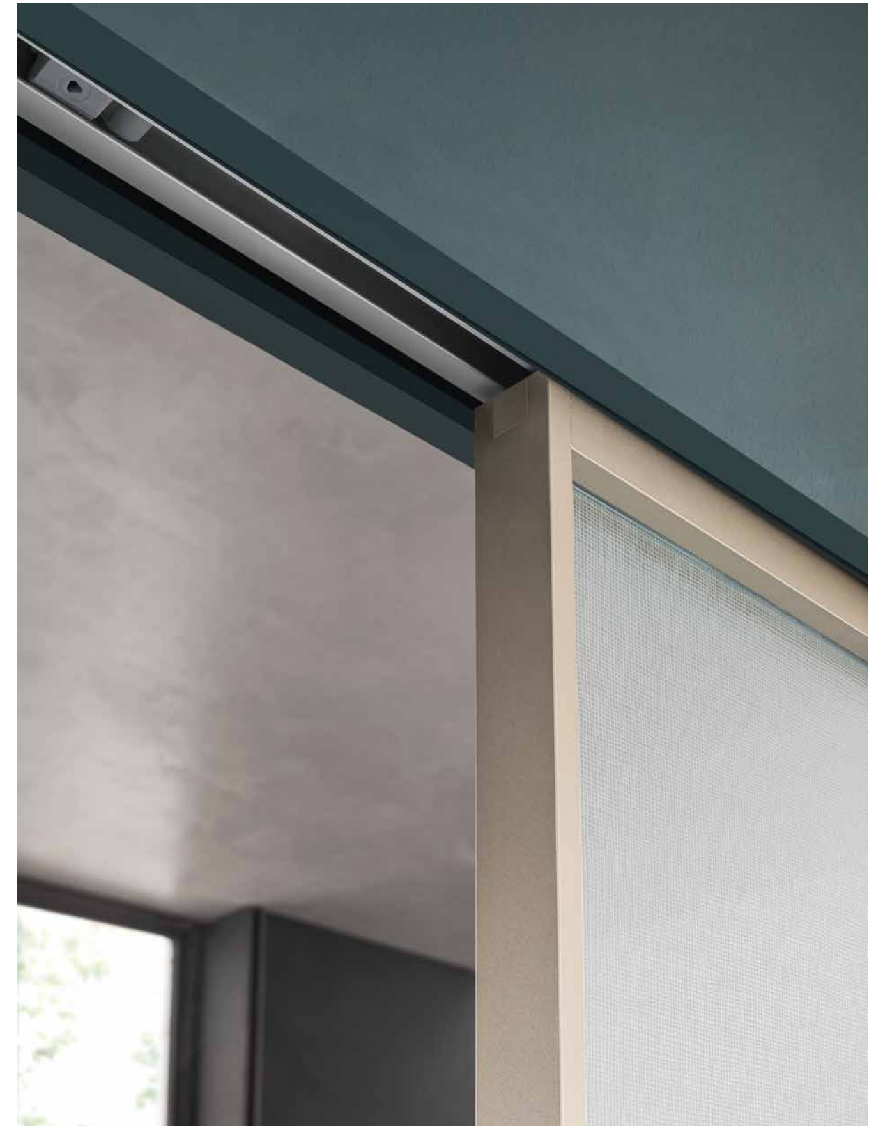
Sistema di scorrimento interno muro Minima Sliding door system inside the wall Minima
