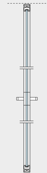
Bilico Senza stipite Without jamb
