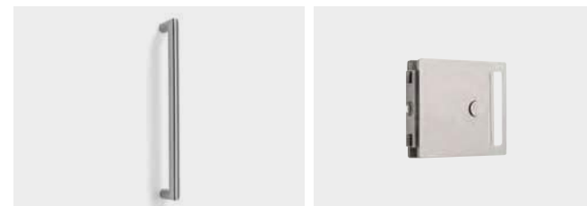
R-10 Il modello R10 è disponibile: R10 handle is available: Ø25x300 - Ø25x650 - Ø30x1000
