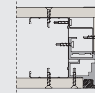
Cartongesso Plasterboard
