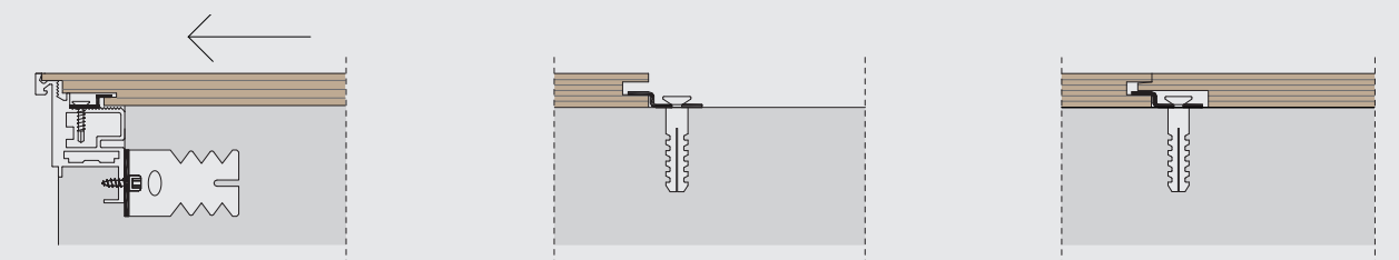
Installazione pannello iniziale Installation of the starting panel
