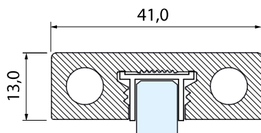
MONTANTE / Sides
