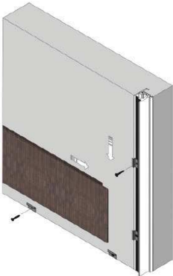
Installazione pannello iniziale Boiserie-H Installation of the starting panel Boiserie-H
